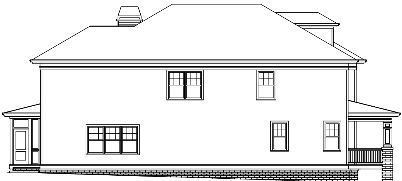
RIGHT ELEVATION
